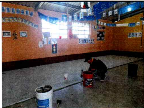
Foto 9: Proceso de colocación de piso de granito en módulo de aulas.
